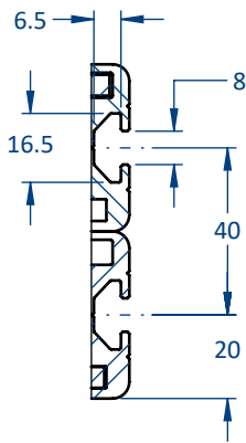
COUPE A-A SCALE 1 : 2 MOUNTING : T-NUT 8MM SLOT M6
